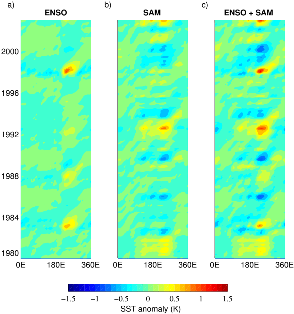
FIG. 10. Time-longitude diagrams, showing the SST simulated from the heat fluxes regressed on a) Niño3, b) SAM, c) Niño3 + SAM.
